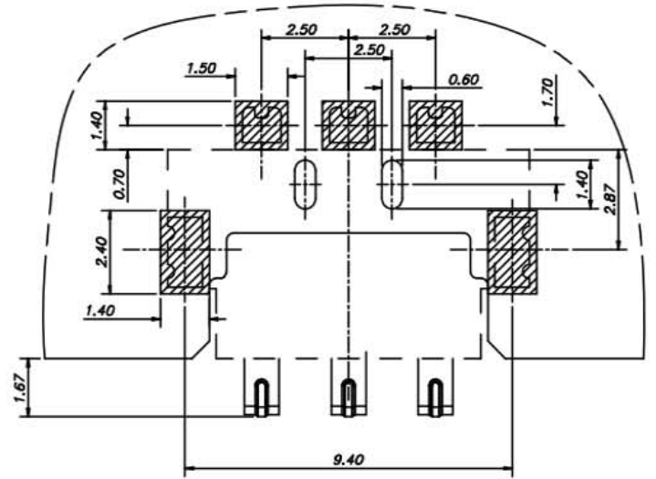
PCB布线图 未注尺寸公差: ±0.05
