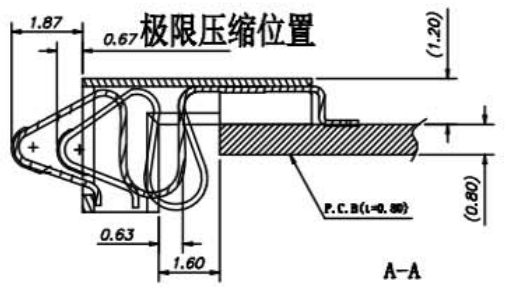
剖视图
