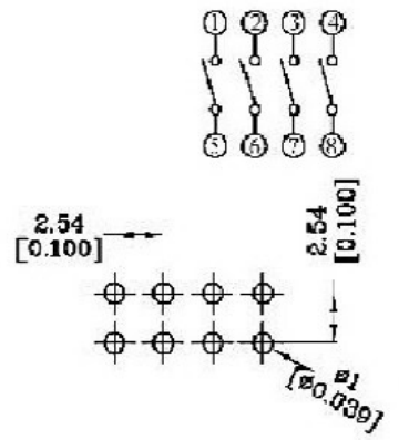
P.C.B LAYOUT
