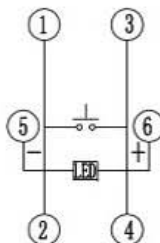
电原理图
