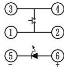
电原理图
