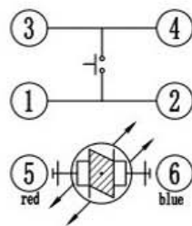
电原理图
