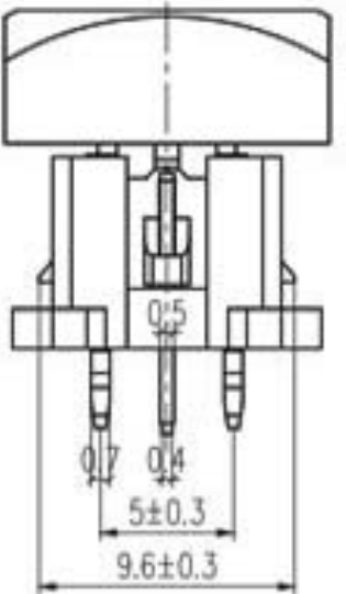
A向
