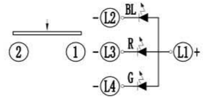
电原理图
