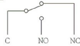
电路简图
