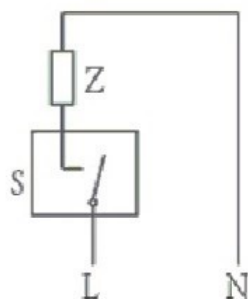
电路简图
