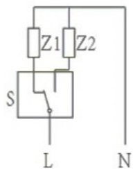
电路简图
