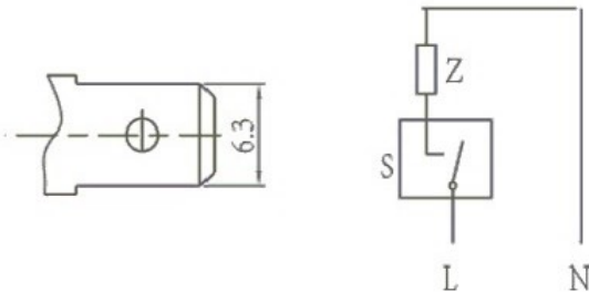
电路简图
