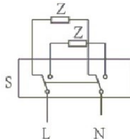
电路简图
