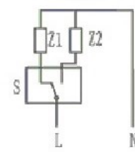
电路简图
