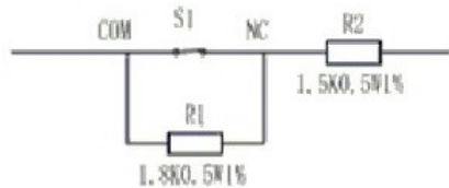
电路简图
