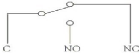
电路简图
