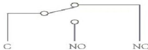
电路简图
