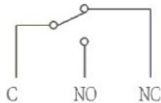
电路简图
