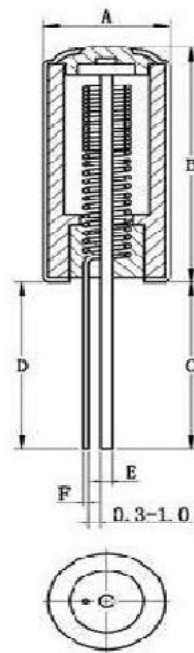
密封式
