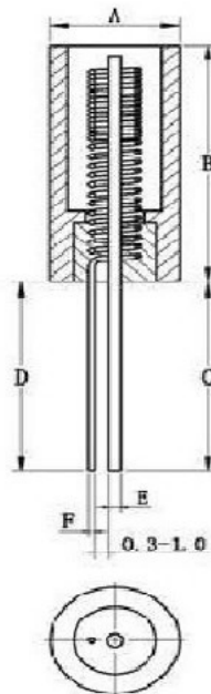
不密封式
