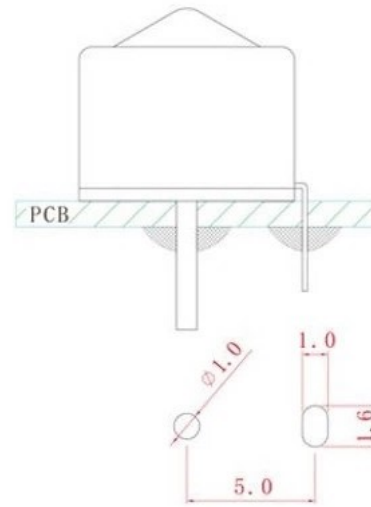
PCB焊锡插脚孔位
