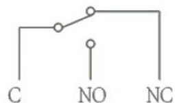
电路简图
