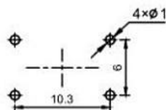
P.C.B. LAYOUT
