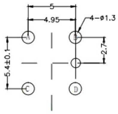
安装尺寸
