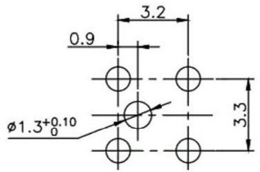
PCB安装尺寸
