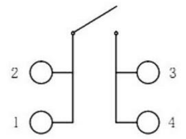
电路图
