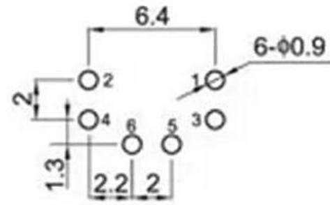
印制电路板 printed-circuit board
