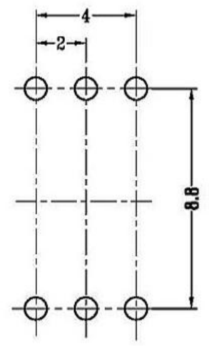
P.C.B LAYOUT TOP VIEW 注：“*”表示关键尺寸(3个).
