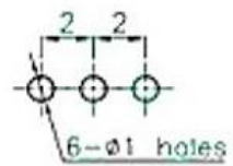
PCB Layout(Pattern Side)
