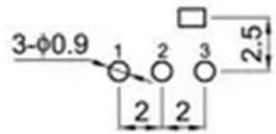
印制电路板 printed-circuit board
