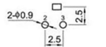
印制电路板 printed-circuit board
