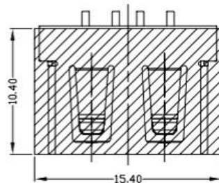
MYLAR 示意图
