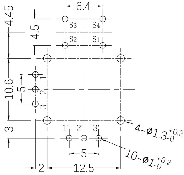
PCB板尺寸图
