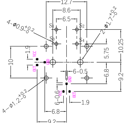
PCB板尺寸图
