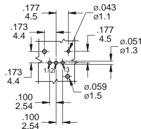
SPDT
