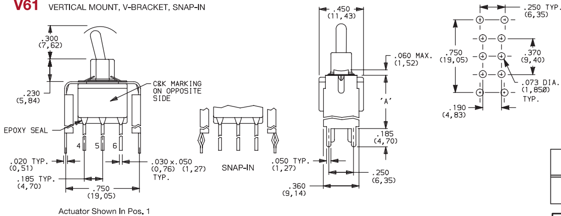
E201MD1_BE DPDT
