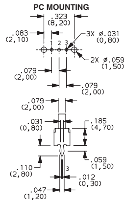
KSD-OS102011MS2QN1 SPDT
