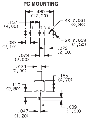
KSD-OS103011MS8QP1 SP3T
