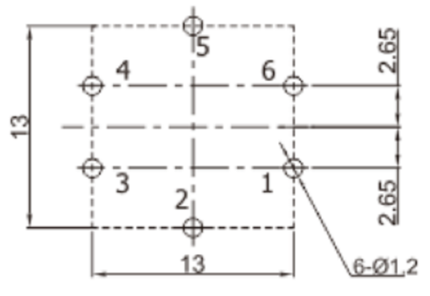
P.C.B.LAYOUT
