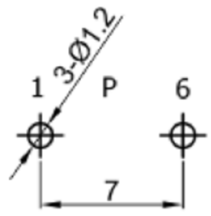
P.C.B. LAYOUT
