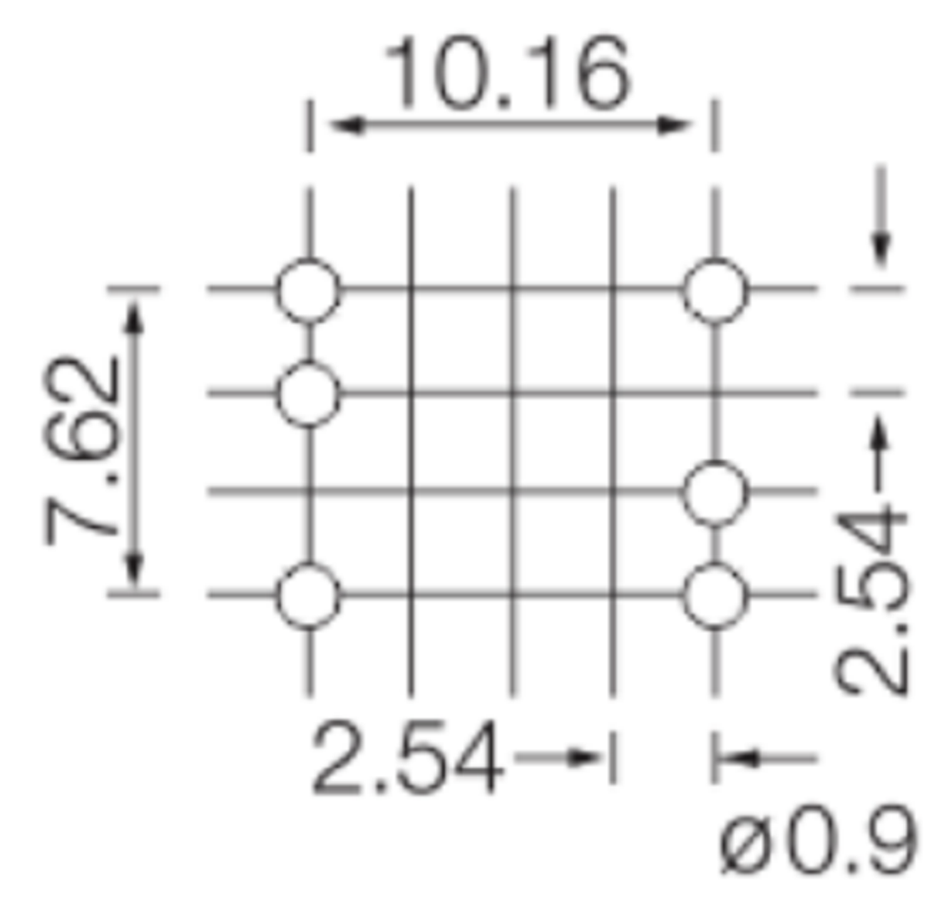
P.C.B Layout
