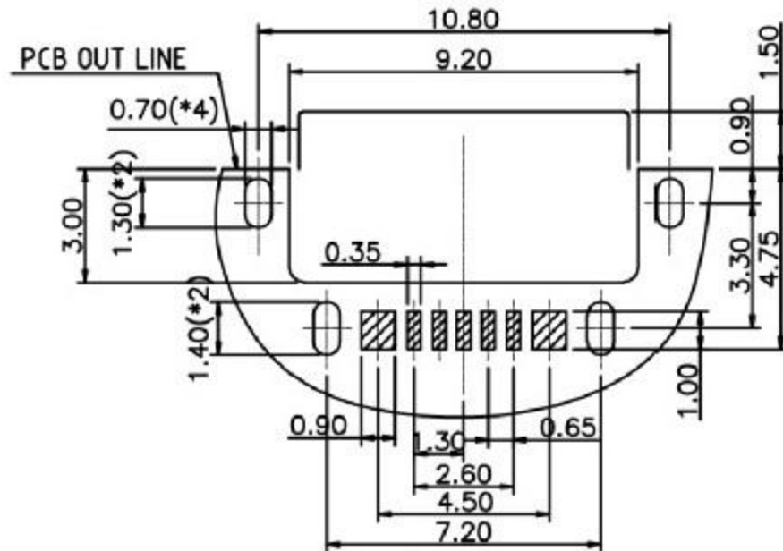
P.C.B LAYOUT
