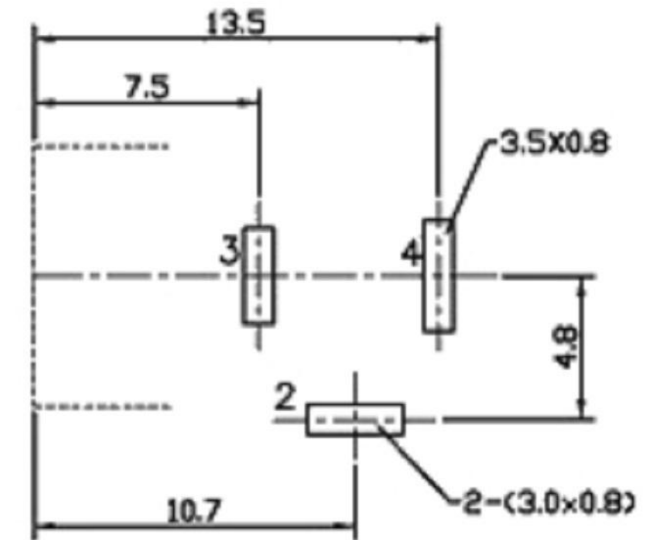
线路板开孔尺寸 P.C.B LAYOUT
