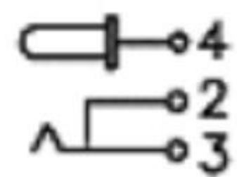
接点示意图 SCHEMATIC
