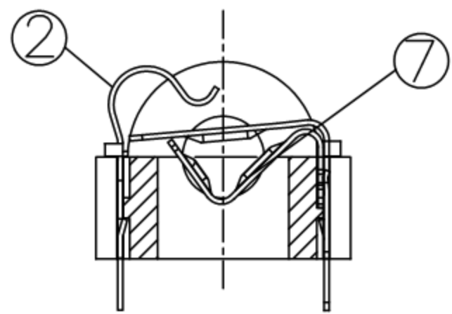
A-A剖面
