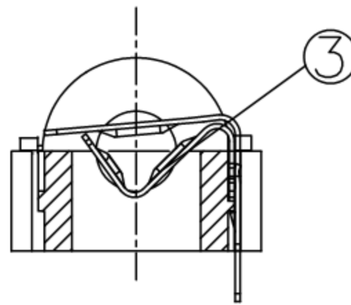
A-A剖面
