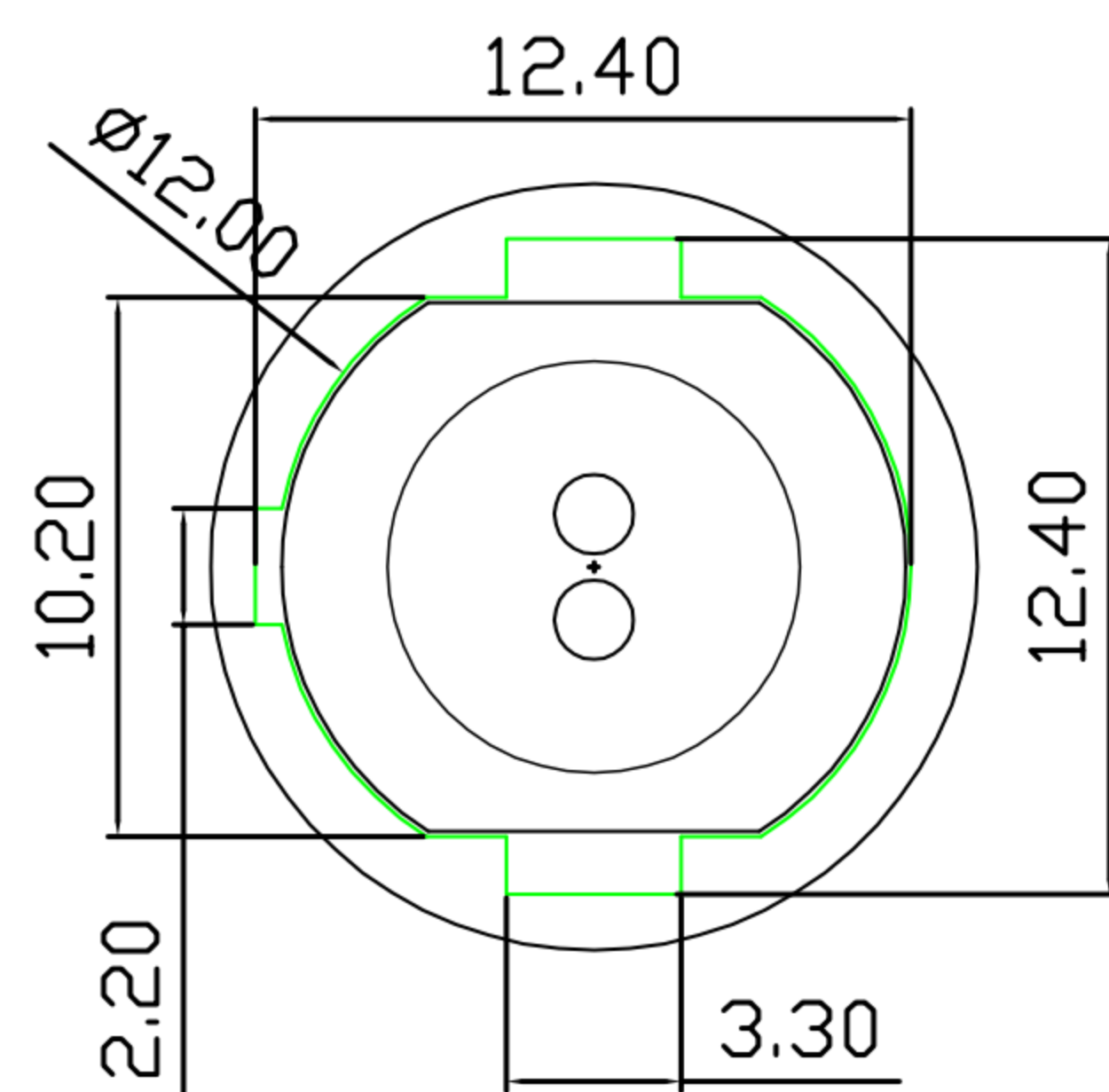
开孔尺寸
