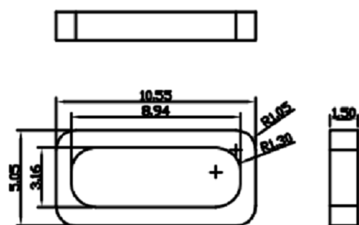
密封圈
