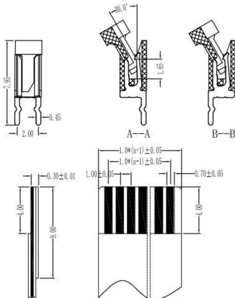
适用扁平电缆
