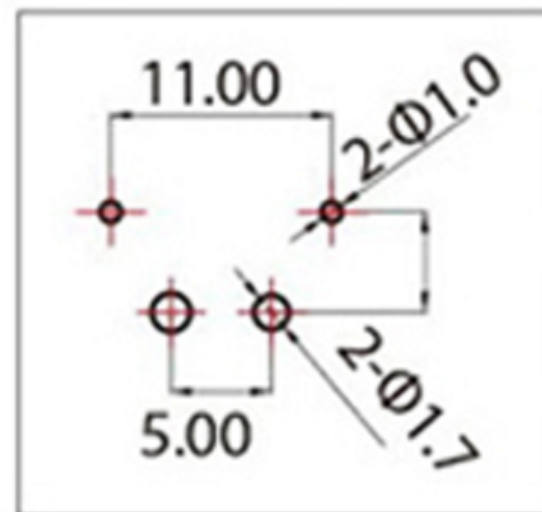
安装孔示意图
