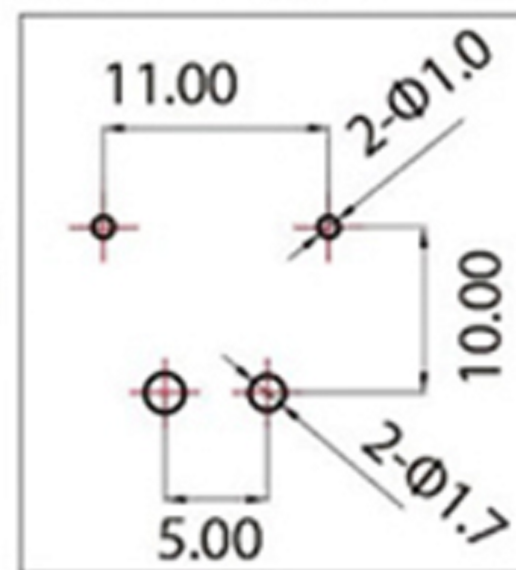
安装孔示意图
