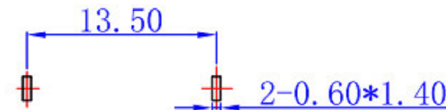
安装孔尺寸示意图
