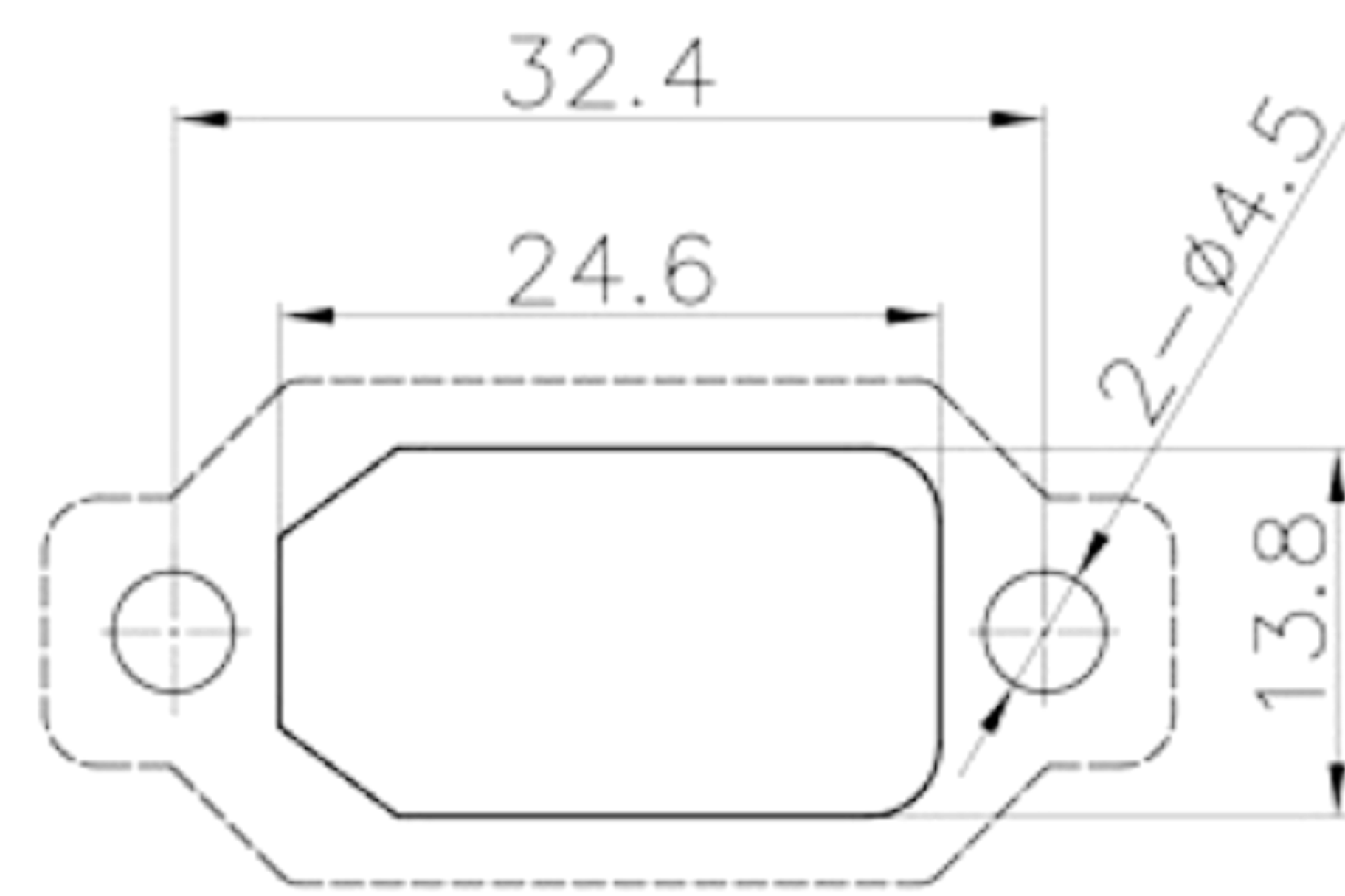
安装孔尺寸
