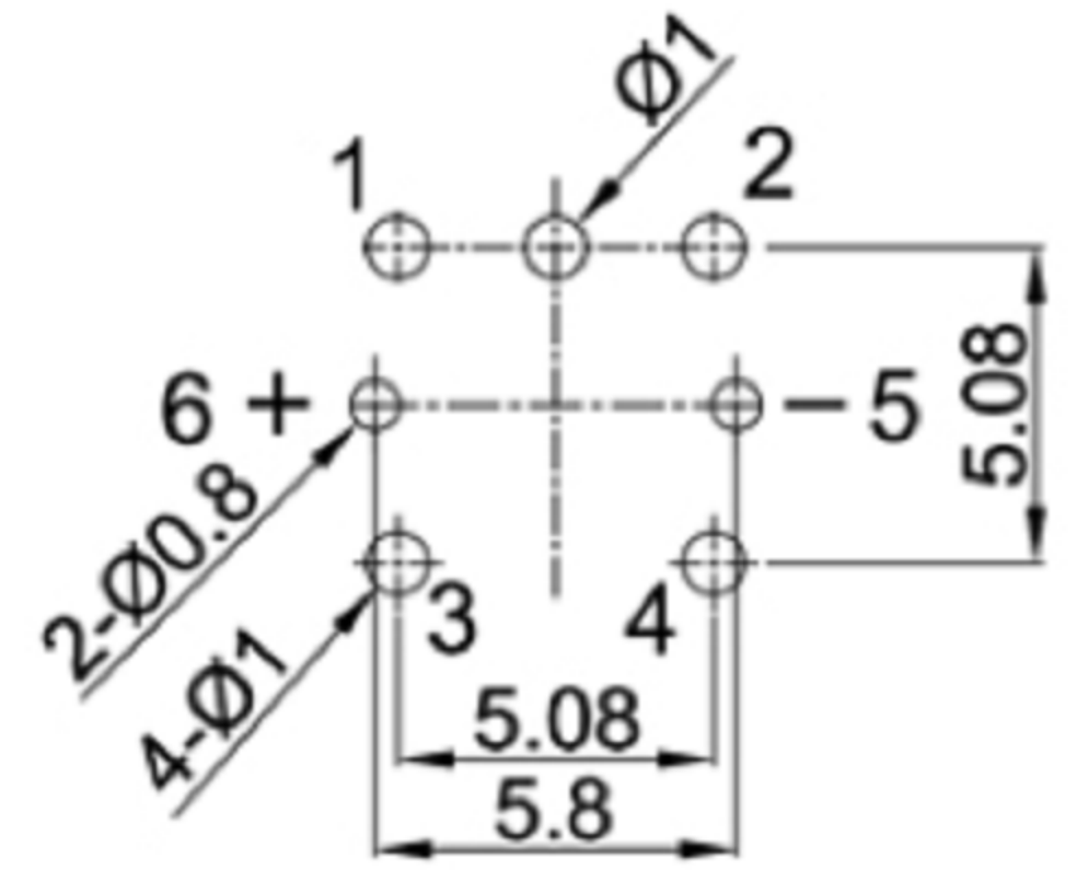
P.C.B. LAYOUT
