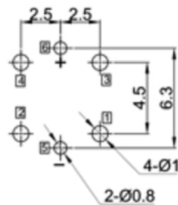
P.C.B. LAYOUT
