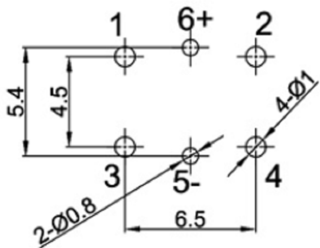
P.C.B. LAYOUT
